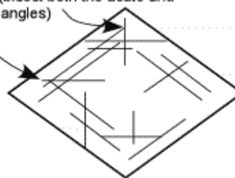
Dolomite
