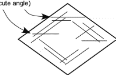
Calcite
